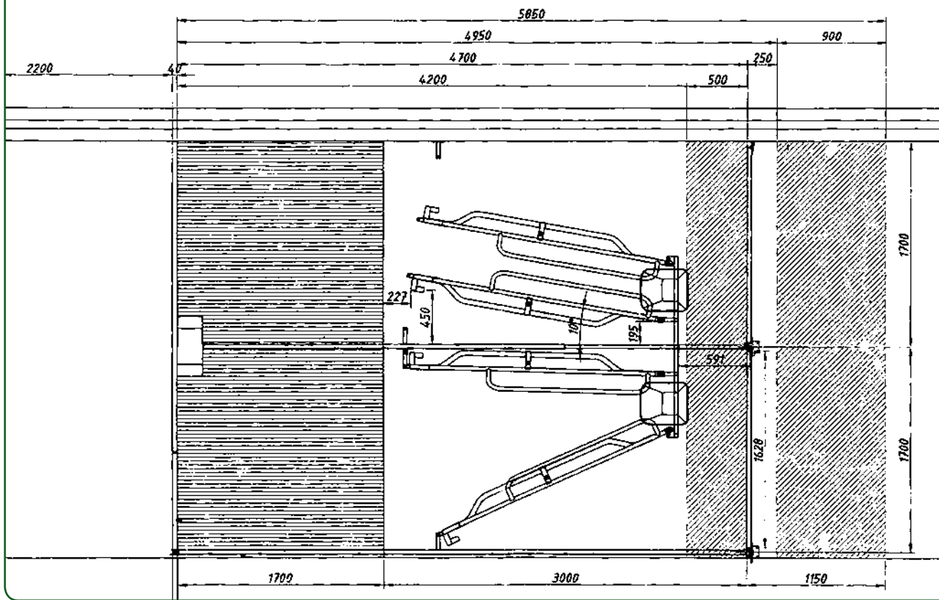
Bovenaanzicht kraamstal
